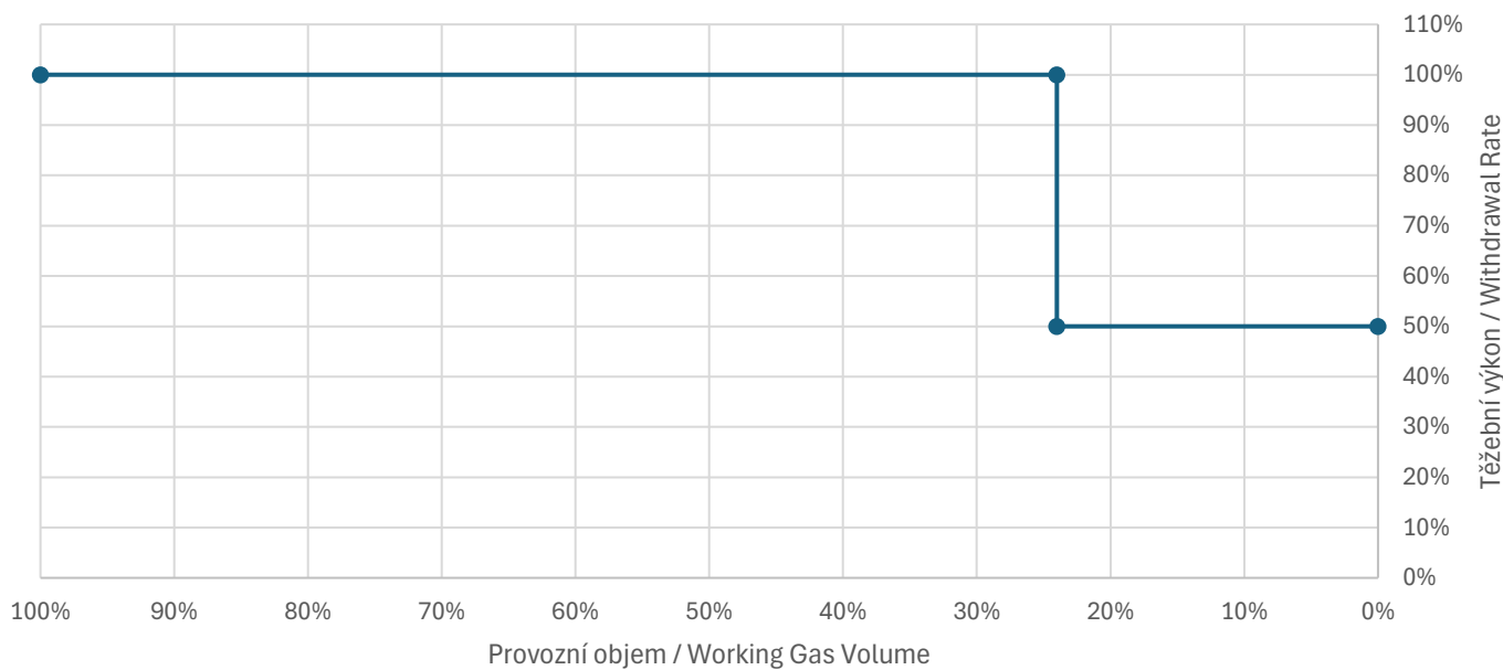
Těžeční křivka / Withdrawal Curve
